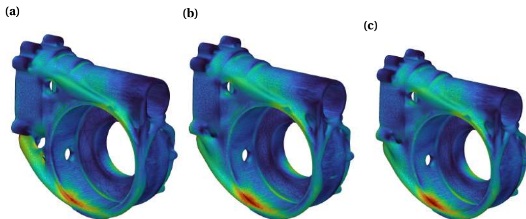
Rys. 8.20. Naprężenia w korpusie pod wpływem obciążenia \alpha = 45^\circ dla różnych przypadków obciążeń: a - 4, b - 8, c - 16
